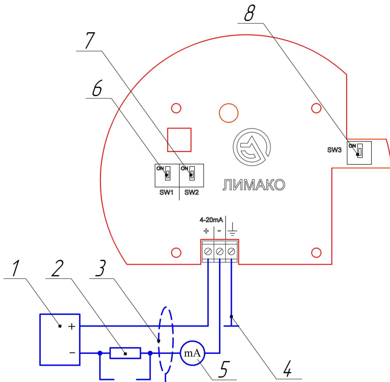
Рис. 5.8 Подключение уровнемера модификации УЛМ-31А1-НF-F-LC. Двухпроводное исполнение.
