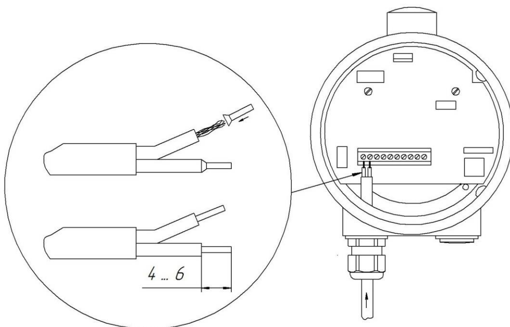
Рис. 5.12 Подключение уровнемера.
