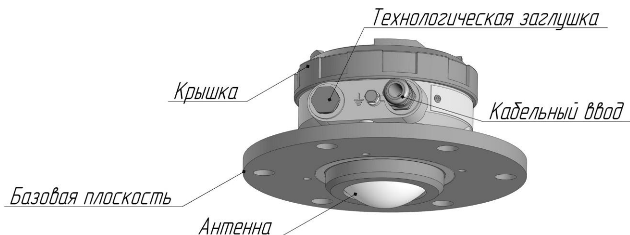
Рис. 3.1. Внешний вид и расположение основных элементов уровнемера УЛМ-31-НФ, УЛМ-31А1-НФ.
