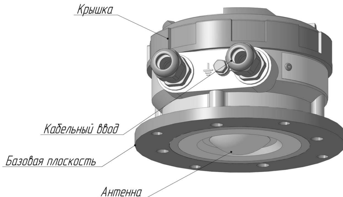
Рис. 3.3. Внешний вид и расположение основных элементов уровнемера УЛМ-31-HF-F, УЛМ-31A1-HF-F и УЛМ-31A1-HF-F-LC. Алюминиевый корпус.
