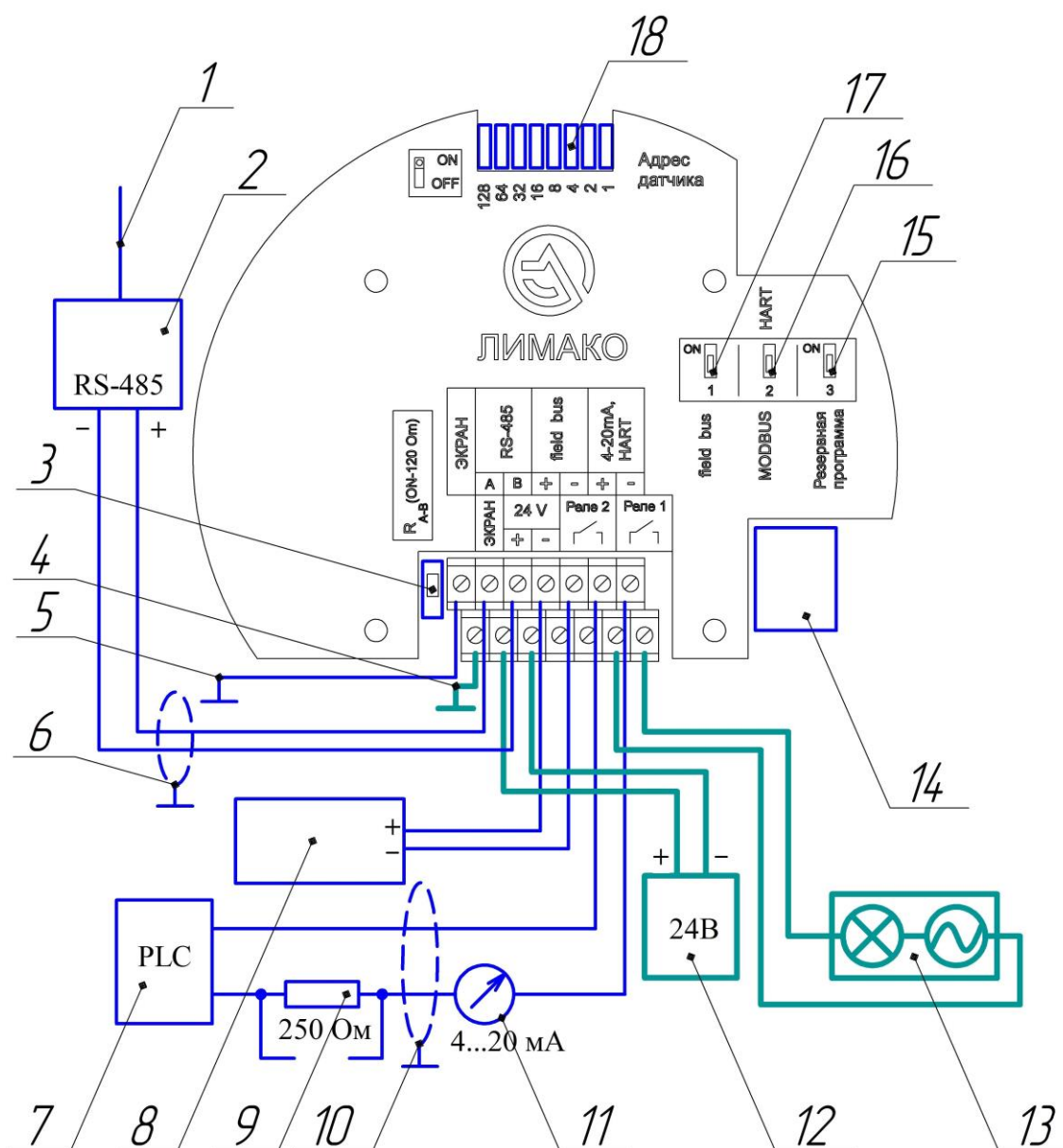
Рис. 5.5 Подключение уровнемеров УЛИМ-31А1, УЛИМ-31-НФ, УЛИМ-31-НФ-Ф, УЛИМ-31А1-НФ и УЛИМ-31А1-НФ-Ф. Вариант 3.
