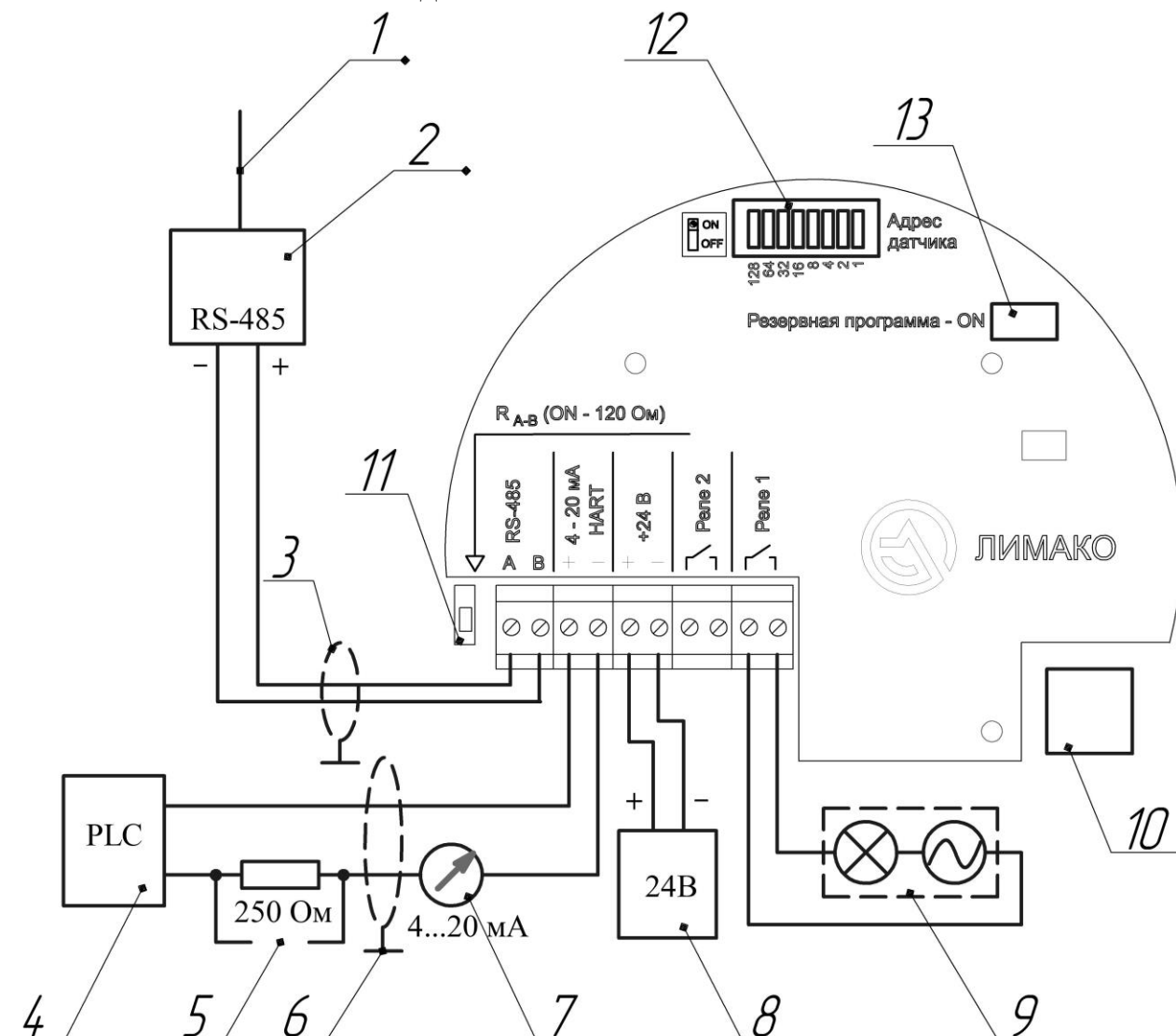
Рис. 5.3 Подключение уровнемеров УЛМ-31А1, УЛМ-31-НФ, УЛМ-31-НФ-Ф, УЛМ-31А1-НФ и УЛМ-31А1-НФ-Ф. Вариант 1.
