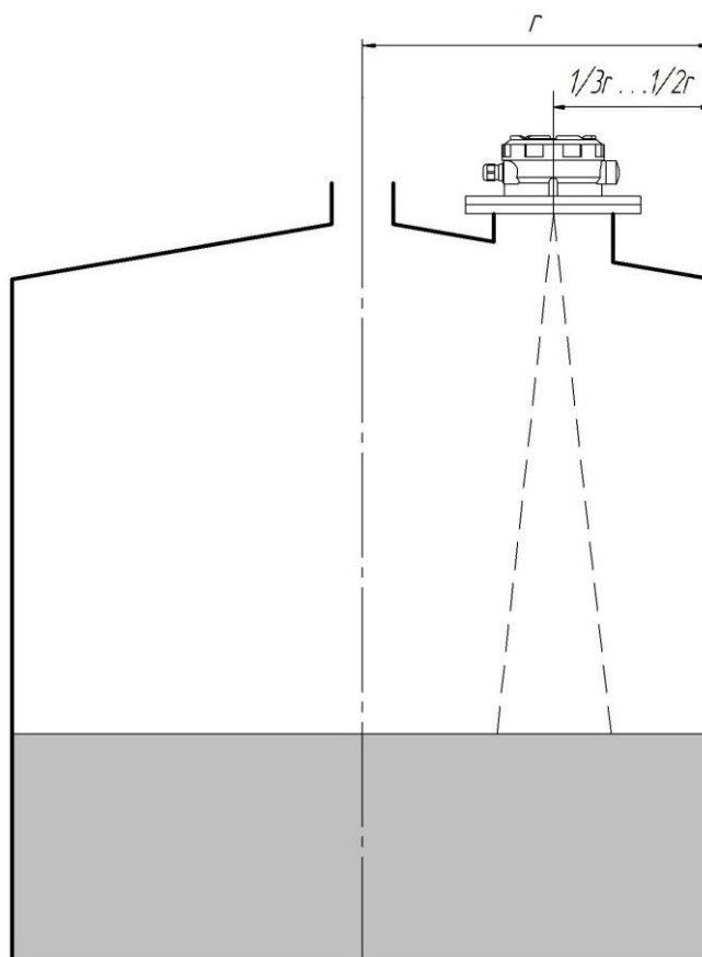
Рис. 4.7. Установка прибора
