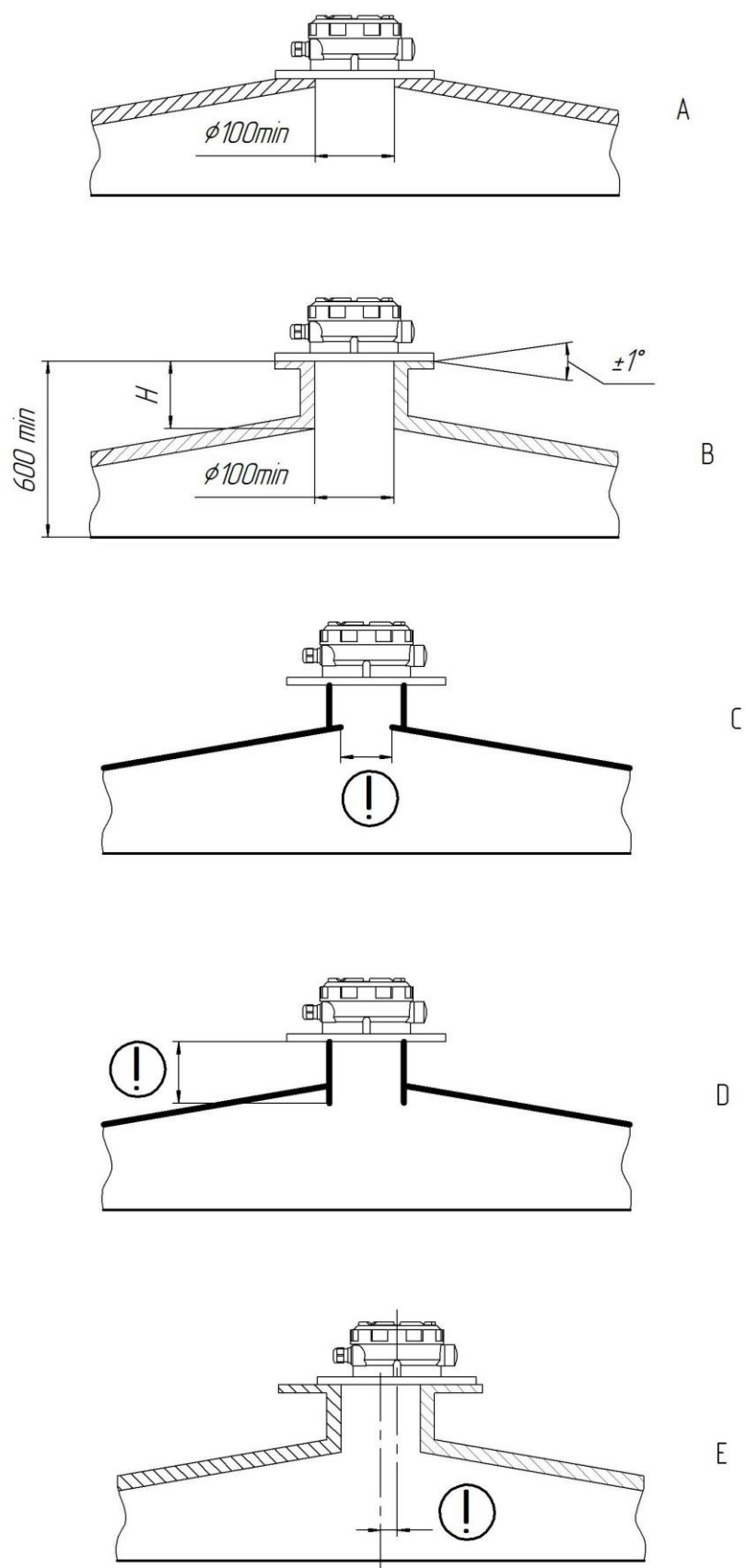
Рис. 4.12. Примеры монтажа
