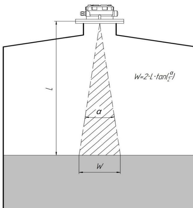
Рис. 4.10. Зона действия измерительного луча
