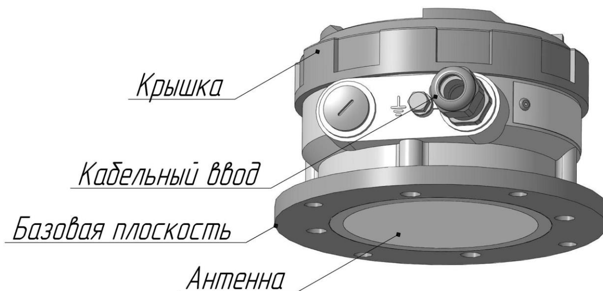
Рис. 3.2. Внешний вид и расположение основных элементов уровнемера УЛМ-31А1.
