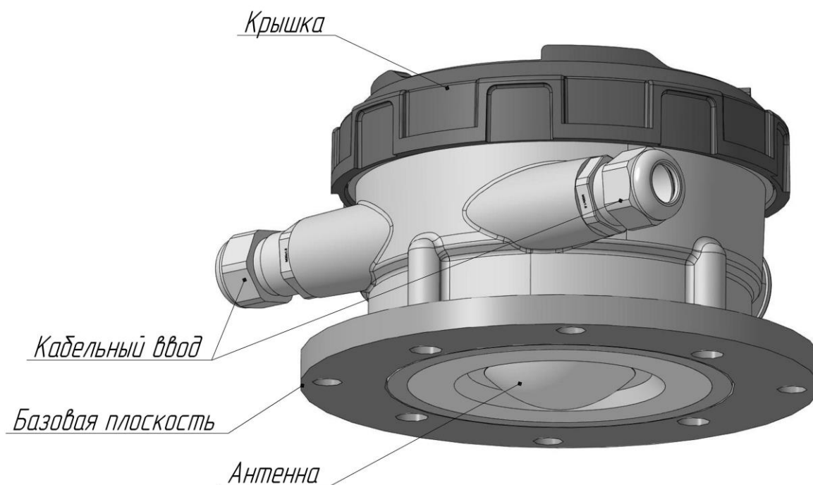
Рис. 3.4. Внешний вид и расположение основных элементов уровнемера УЛМ-31-HF-F, УЛМ-31A1-HF-F и УЛМ-31A1-HF-F-LC. Пластиковый корпус.
