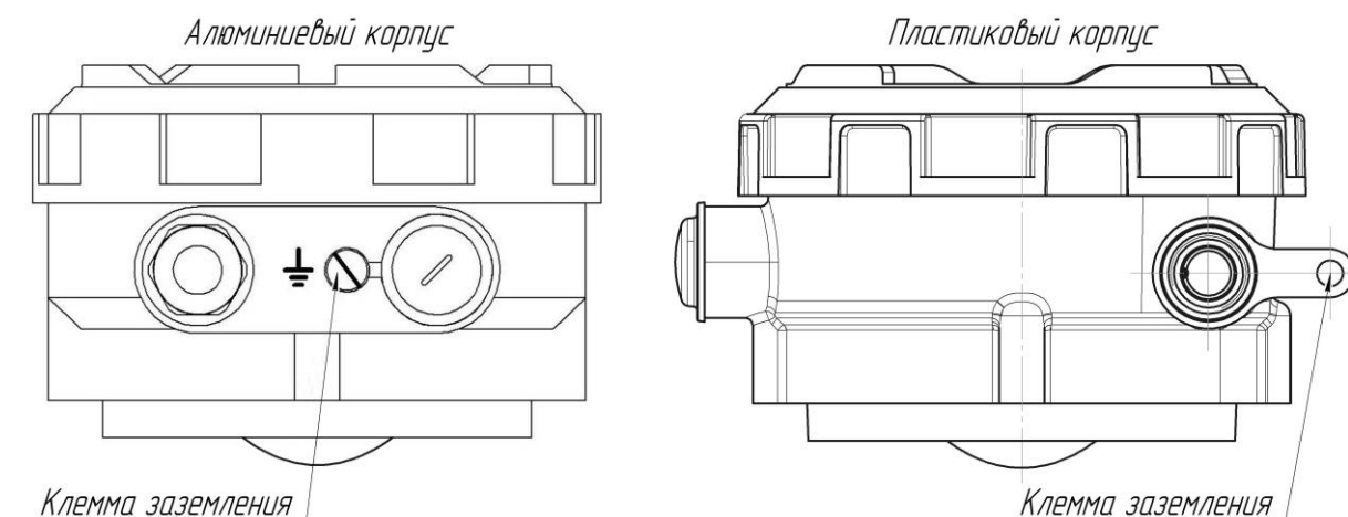
Рис. 5.2 Клемма заземления
