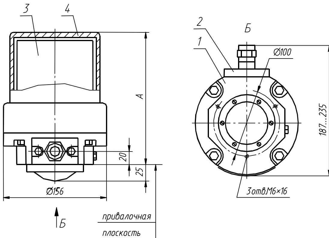
Рис.5.1. Общий вид датчика УЛМ4.01.000, УЛМ4.01.000-А, УЛМ4.01.000-01, УЛМ4.01.000-01-А, УЛМ4.01.000-02, УЛМ4.01.000-02-А.
