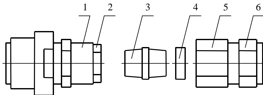
Рис.8.6. Кабельный ввод для бронированного кабеля
